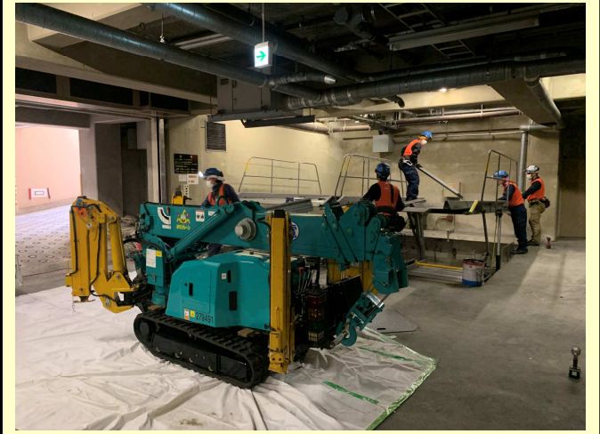
2.9tカニクレーン(3t車搬入)
